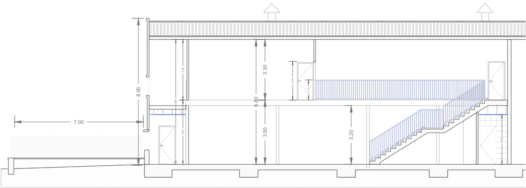
SECCIÓN A-A' e: 1/100
