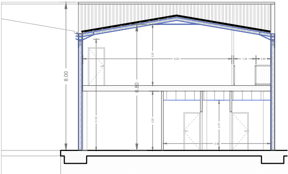
SECCIÓN D-D' e: 1/100
