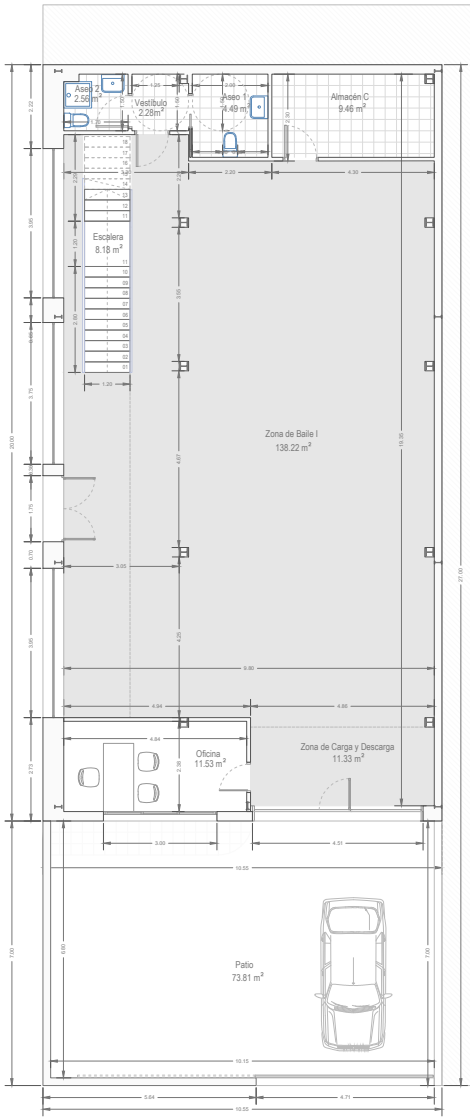
PLANTA BAJA e: 1/100
