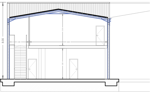
SECCIÓN D-D' e: 1/100
